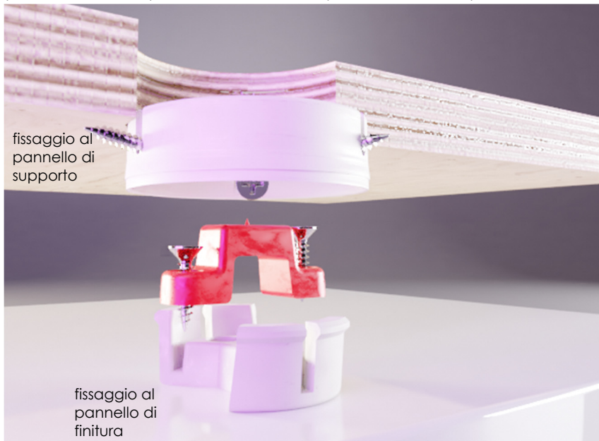
KIT L700904 con resistenza a trazione 16 kg (viti non fornite con il kit)
