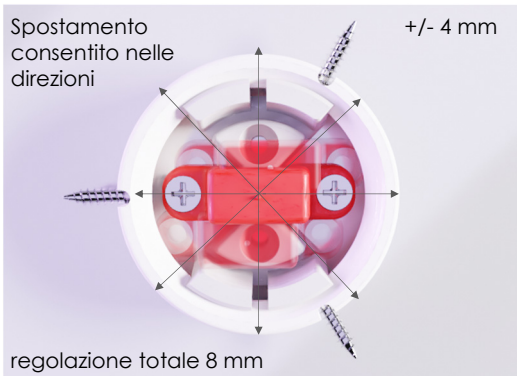
KIT L700905 con resistenza a trazione 8 kg (viti non fornite con il kit)
